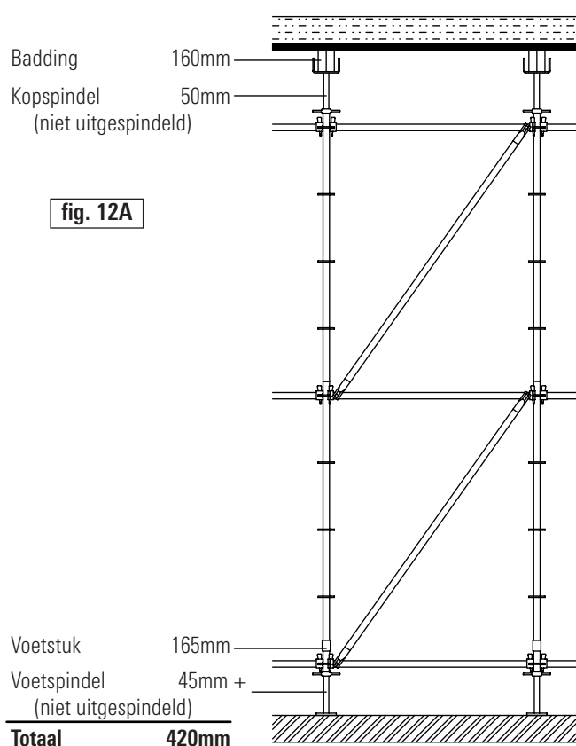
fig. 12: Ondersteuning breedplaatvloer
