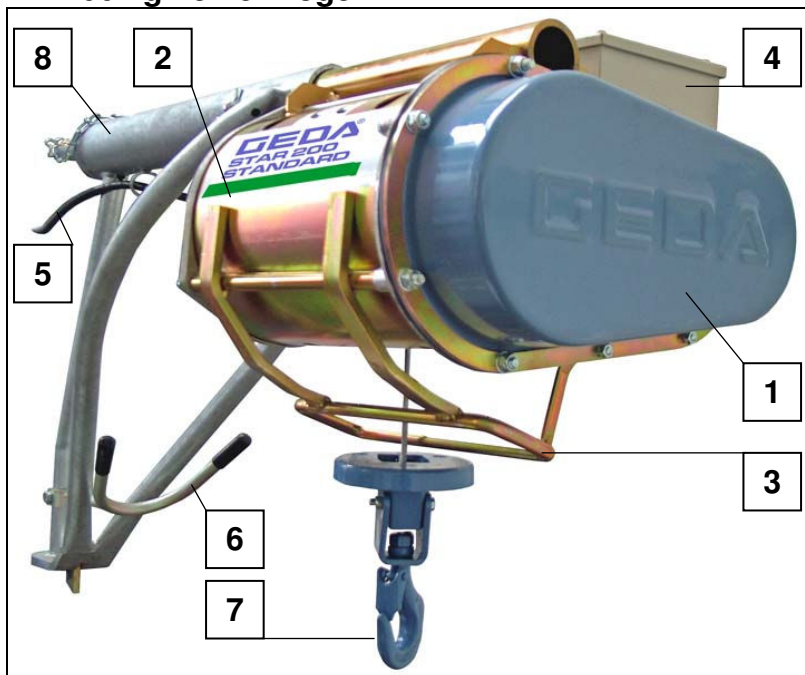
Fig. 3 GEDA STAR 200 STANDARD
