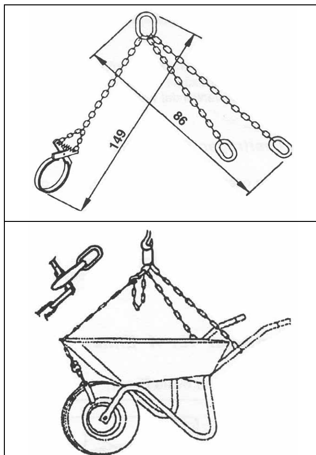
Fig. 20 Kettinghangwerk voor kruitwagen
