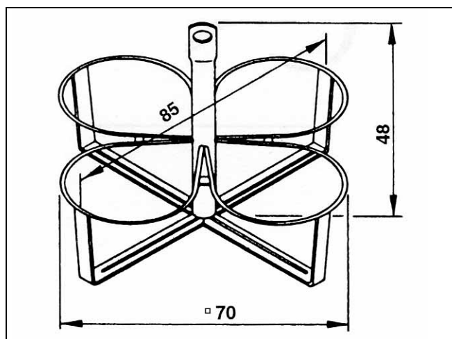
Fig. 15 Emmerdrager voor 4 emmers
