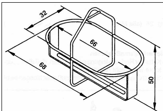
Fig. 14 Emmerdrager voor 2 emmers
