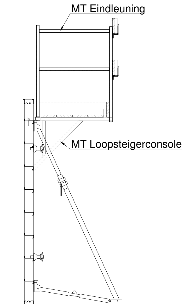
Aanzicht samengestelde Manto kist
